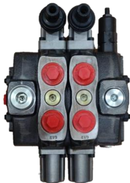
STP-7009 SD8/2 [6 Hole] [2 lever]
